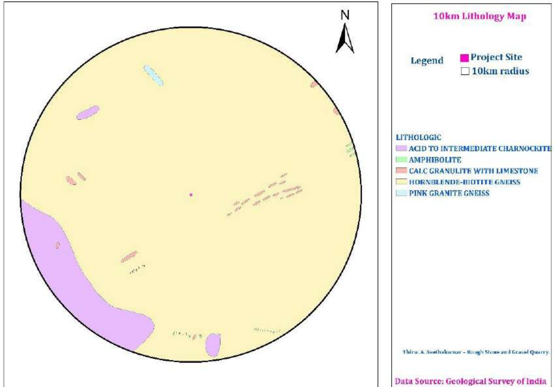
படம்:-2.8..லித்தாலஜி
