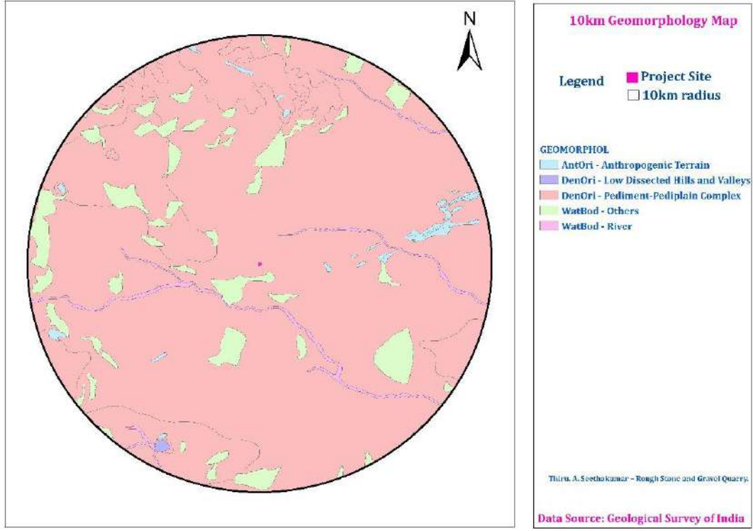
படம்:-2.7..புவி அமைப்பியல்
