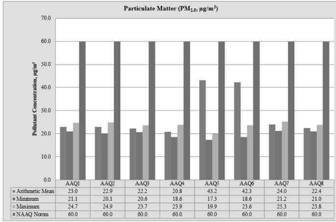
படம் 3.18: காற்றின் தர மாதிரியின் சுருக்க வரைபடம் PM 2.5
