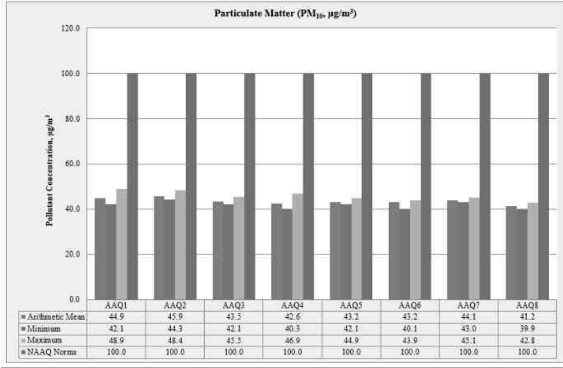
படம் 3.17: காற்றின் தர மாதிரியின் சுருக்க வரைபடம் PM 10
