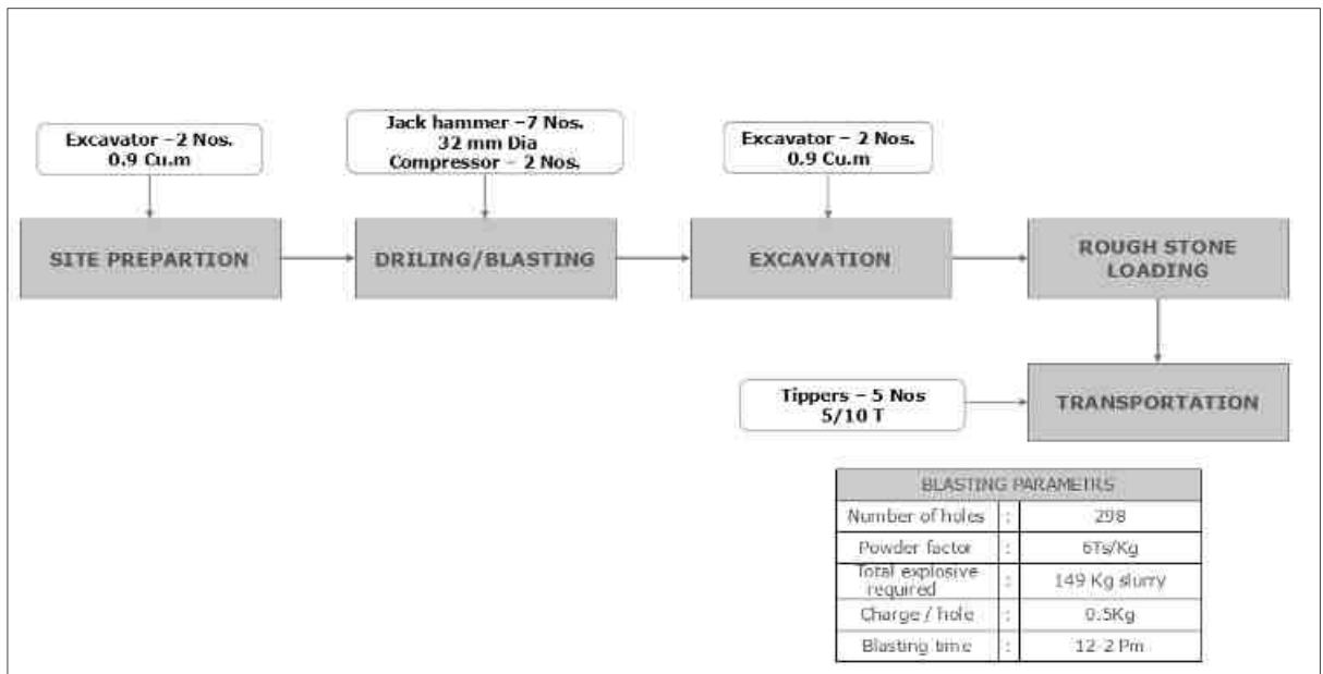
படம் 2.6 செயல்முறை ஓட்ட வரைபடம்
