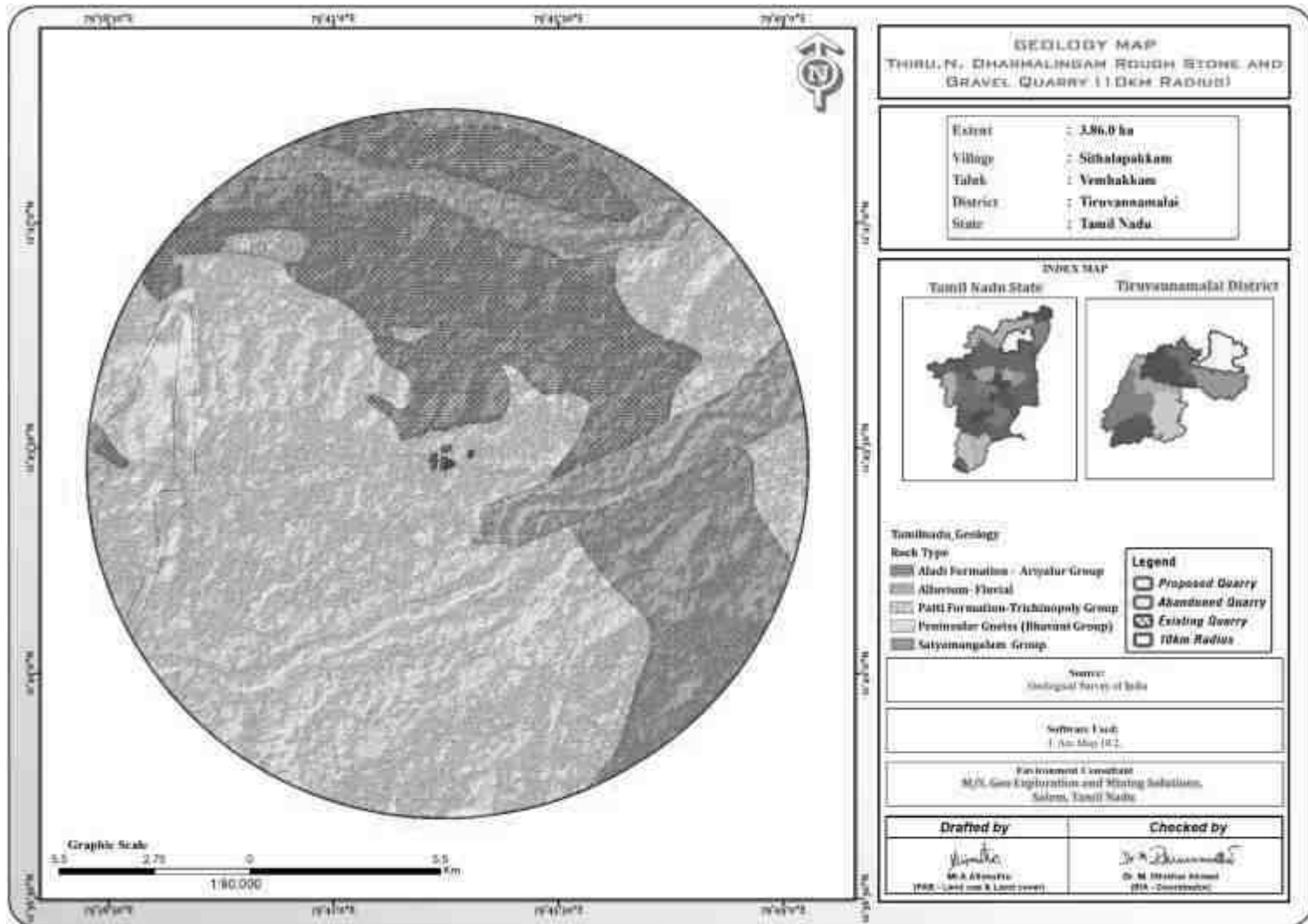
படம் 2.9 மண்டல புனியியல் வரைபடம்
