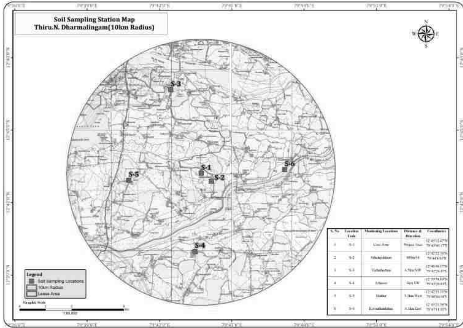
படம் 3.4: 10 கிமீ சுற்றளவில் உள்ள மண் மாதிரி இடங்கள்
