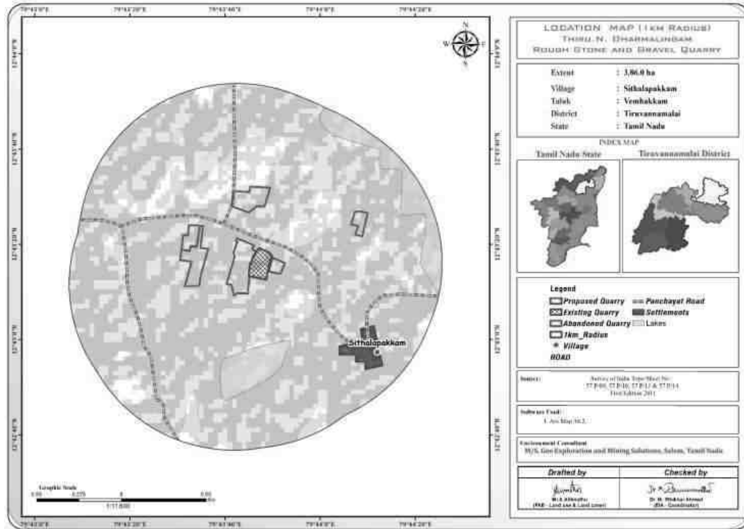
படம் 2.8: 1 கிமீ சுற்றளவில் மேற்பரப்பு வரைபடம்
