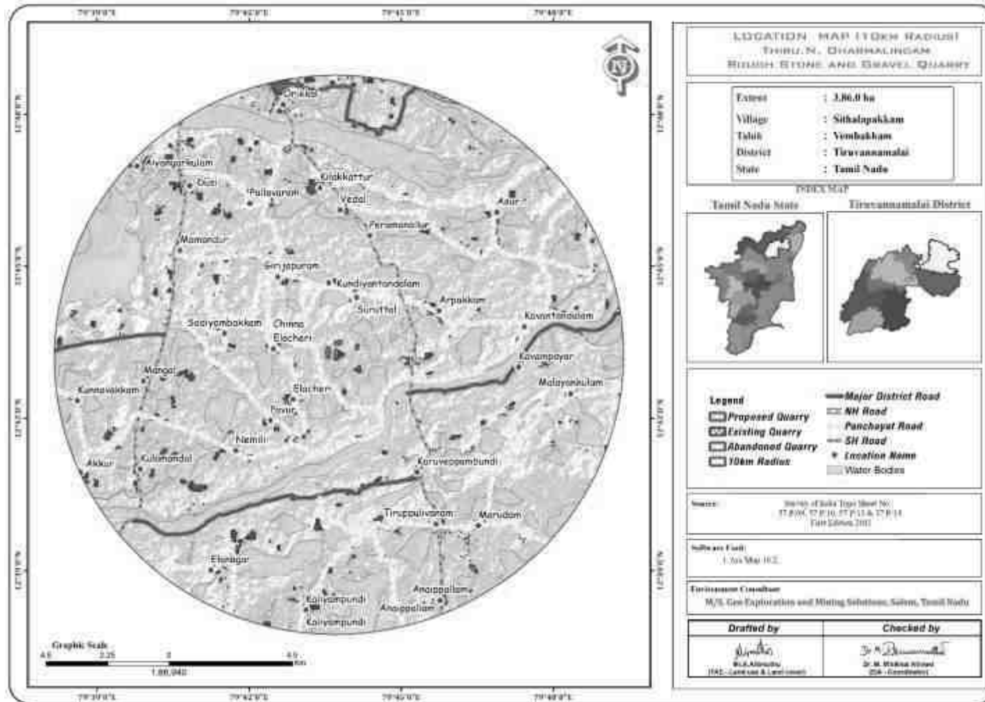
படம் 2.6: 10 கிமீ சுற்றளவைச் சுற்றியுள்ள மேற்பரப்பு வரைபடம்
