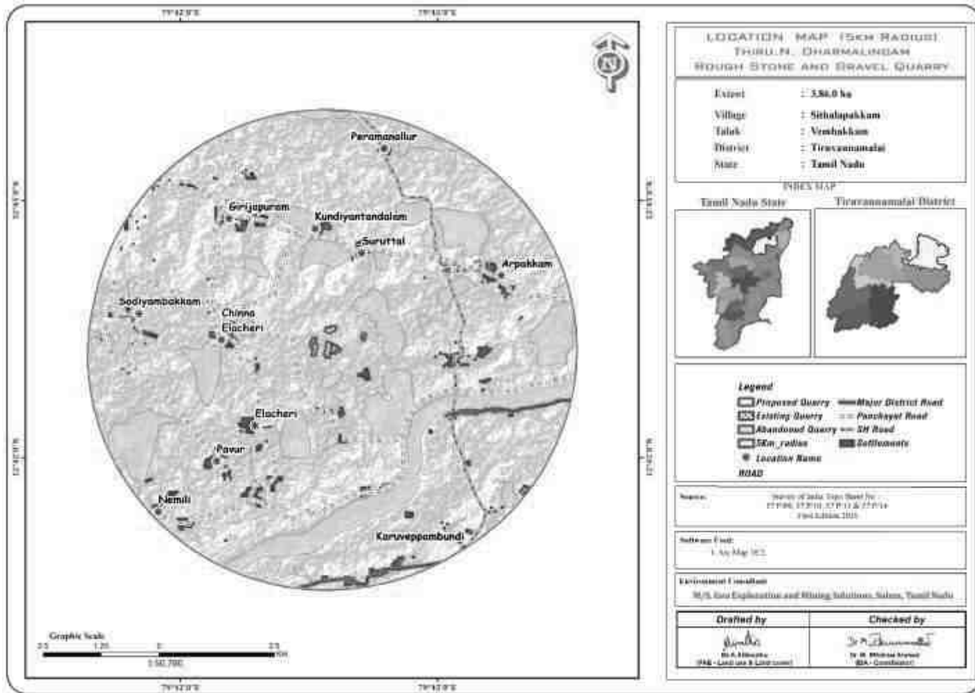
படம் 2.7: 5 கிமீ சுற்றளவைச் சுற்றியுள்ள மேற்பரப்பு வரைபடம்
