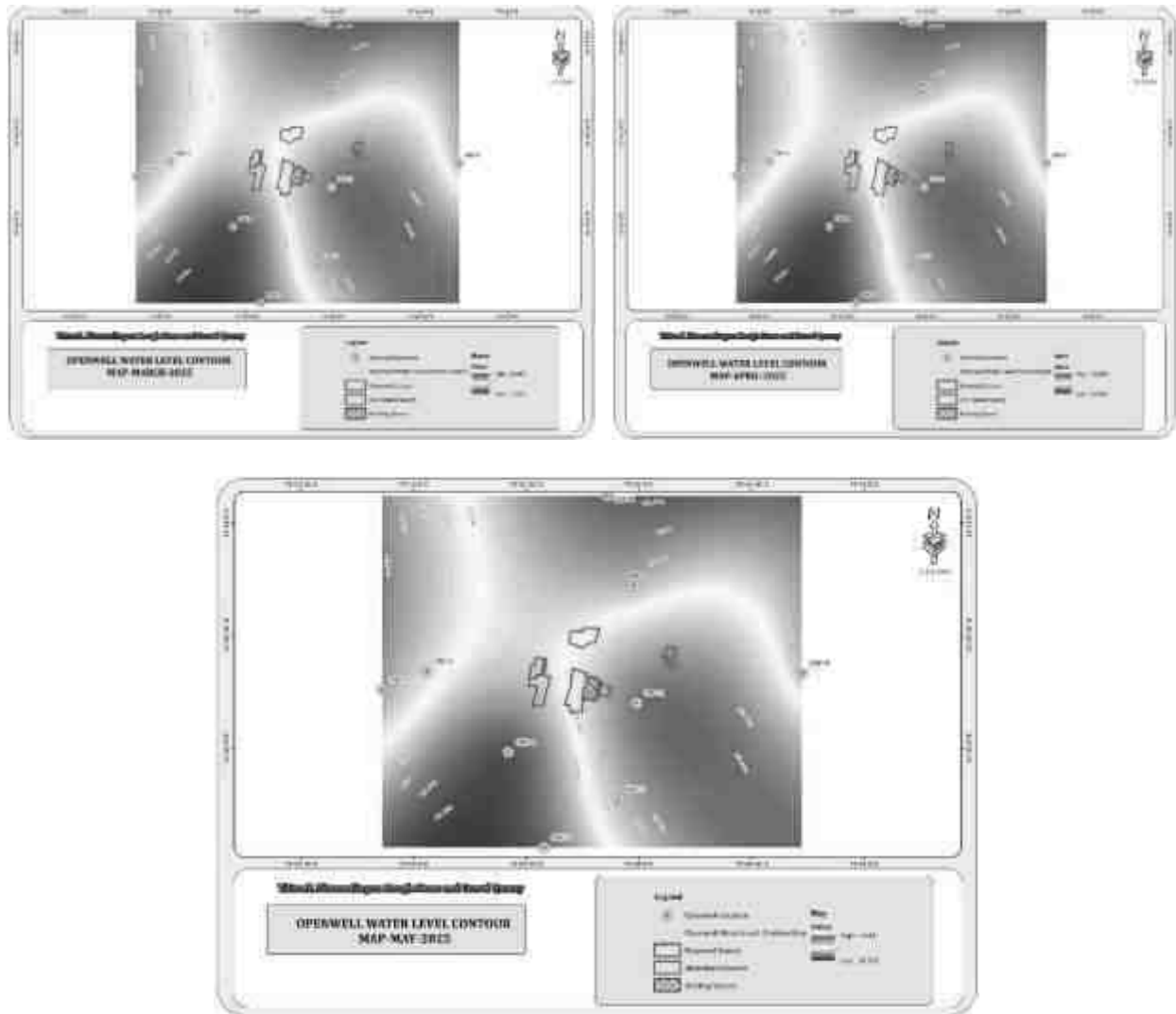
படம் 3.7: திறந்த கிணறு நீர் மட்டத்தின் விளிம்பு வரைபடம் - (மார்ச் முதல் மே 2025 வரை)
