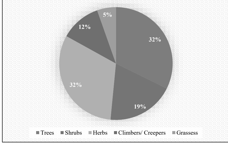
படம் எண். 3.23: தாவர வாழ்க்கை வடிவங்களின் (தாங்கல் மண்டலம்) % விநியோகத்தைக் காட்டும் வரைபடம்.
