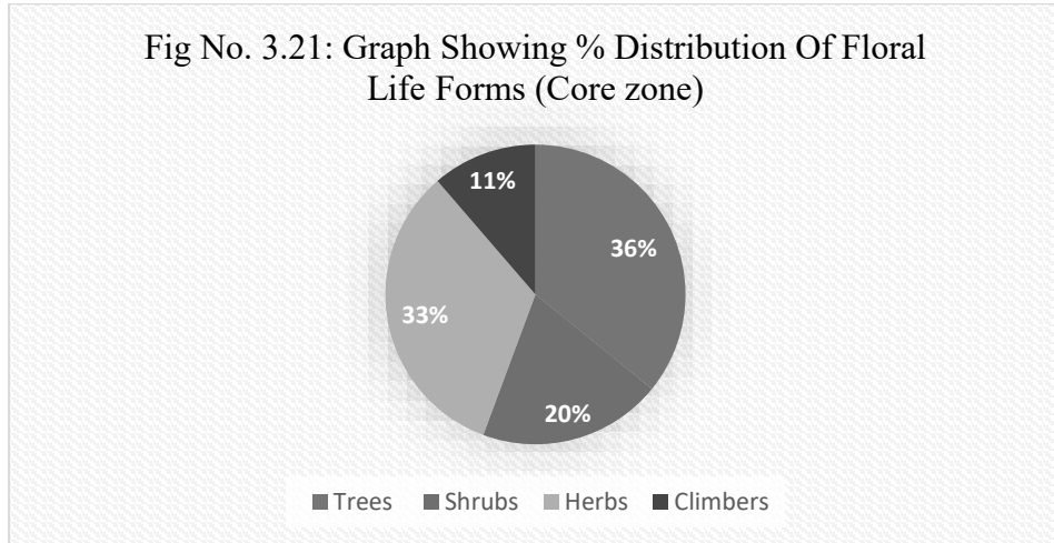
படம் எண். 3.21: தாவர வாழ்க்கை வடிவங்களின் (மைய மண்டலம்) % விநியோகத்தைக் காட்டும் வரைபடம்.
