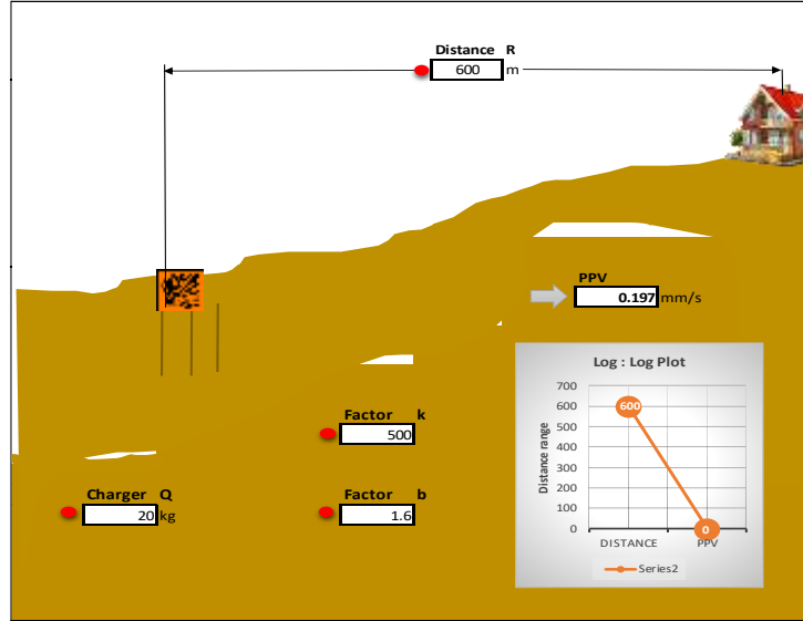
படம் 4.7: நில அதிர்வு கணிப்பு - P2
