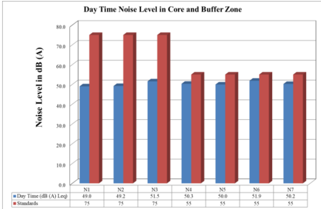
படம் 3.24: மைய மற்றும் இடையக மண்டலத்தில் பகல் நேர இரைச்சல் நிலைகள்
