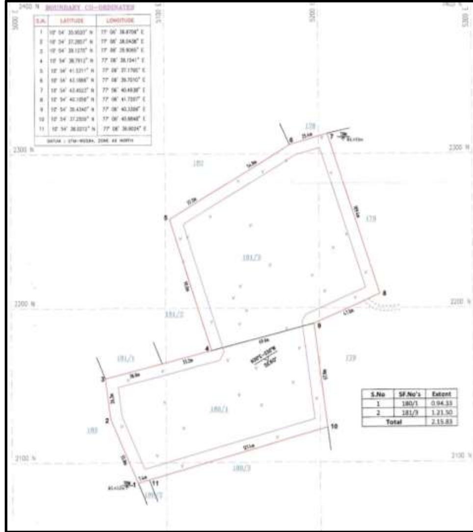
படம் 2.7: குவாரி குத்தகைத் திட்டம் / மேற்பரப்புத் திட்டம் - P1
