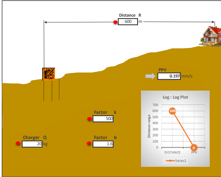
படம் 4.7: நில அதிர்வு கணிப்பு - P2
